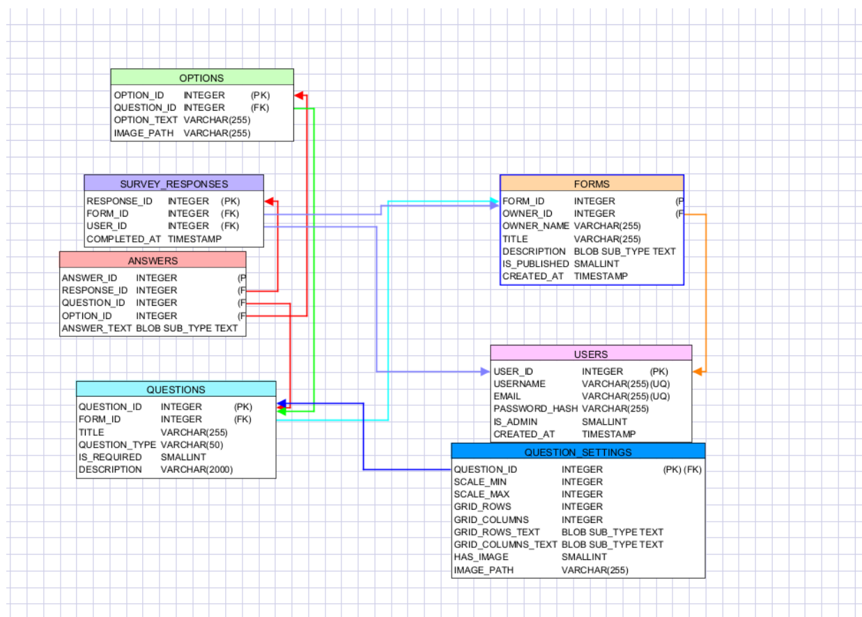
Рисунок 6 – ER-диаграмма
